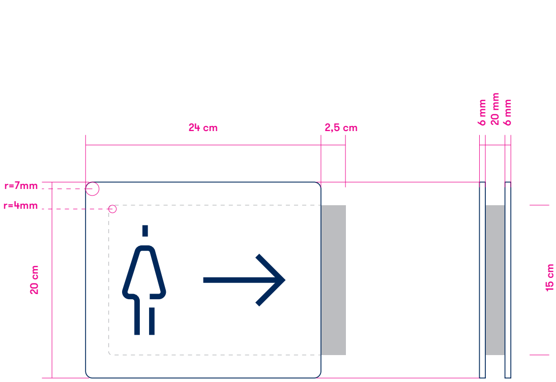
Przekrój
